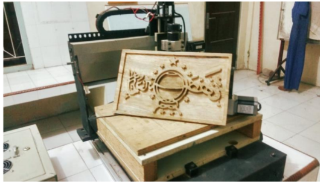
Gambar 11. Proses pembuatan cetakan dengan papan
