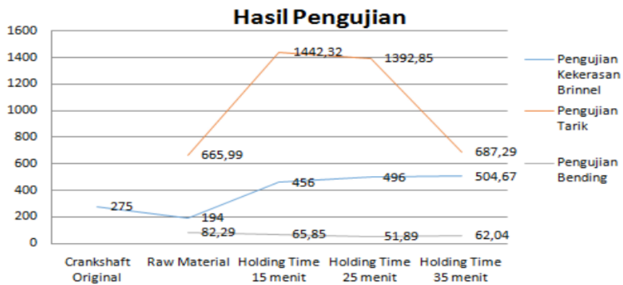
Gambar 6. Pengaruh Variasi Holding Time Terhadap Nilai Kekerasan, Kekuatan Tarik, dan Kekuatan Bending
