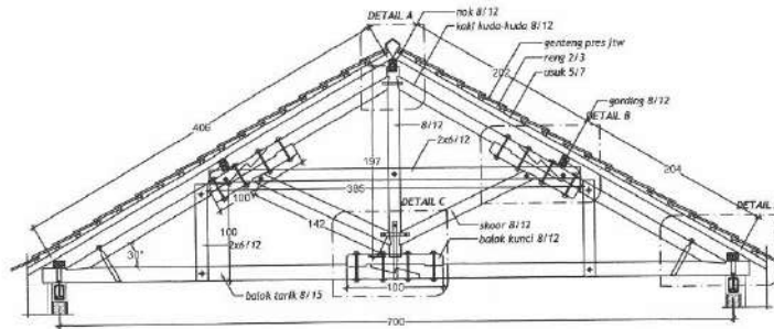
DETAIL KUDA-KUDA (KK2) 1 : 40
